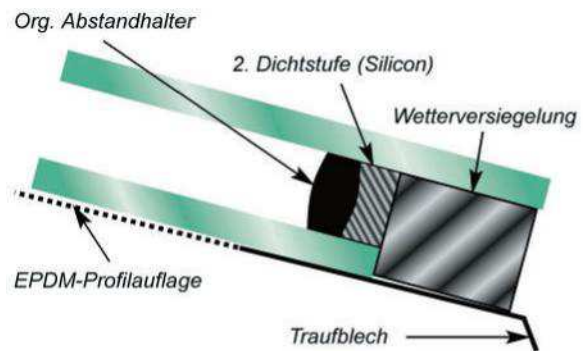
Abb. 3 Fehlerhafte Traufpunktversiegelung
